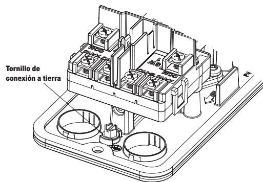
FIGURA 5. UBICACIÓN DEL TORNILLO DE CONEXIÓN A TIERRA
