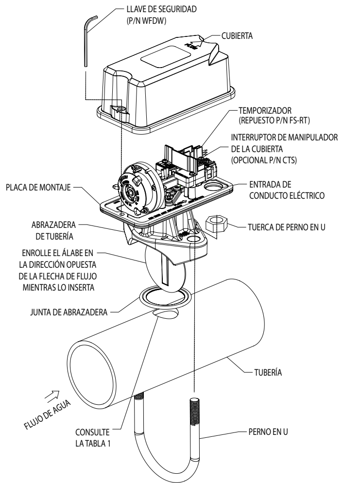
FIGURA 4. DIAGRAMA DE MONTAJE
