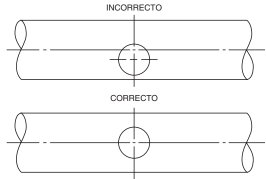
FIGURA 2. UBICACIÓN DEL ORIFICIO DE MONTAJE VISTA SUPERIOR
