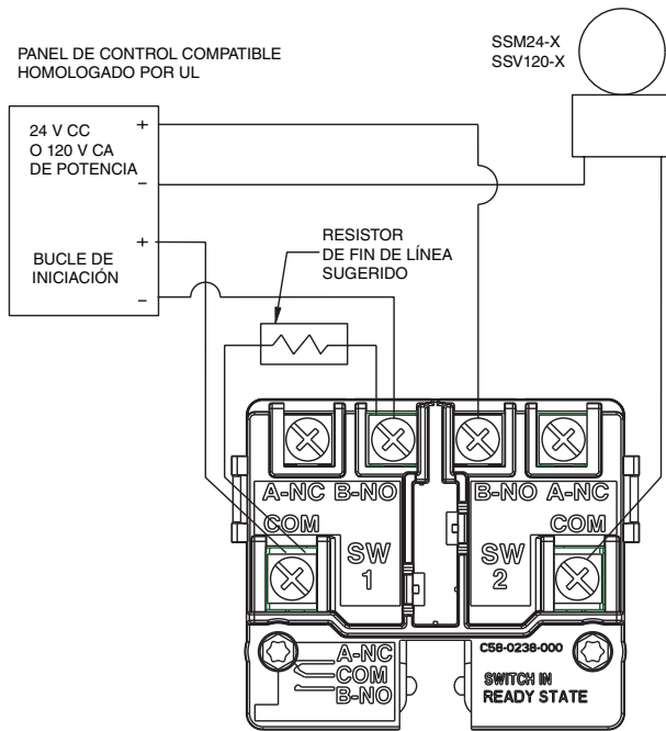
FIGURA 7. CABLEADO DE CAMPO
